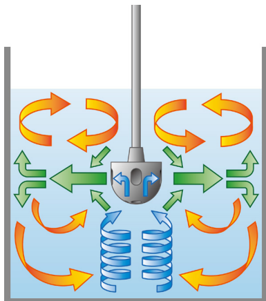
遠心式攪拌の理論図
